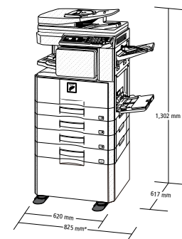
*1 885 mm, když je vyřazena rožň finišerů a pravý výstupní rožň. Obrázek stroje s doplňky.
